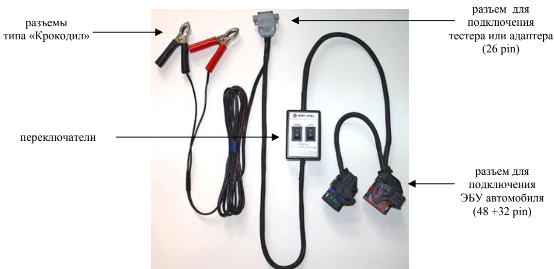
Кабель Д14-K11-M74CAN/K-line
